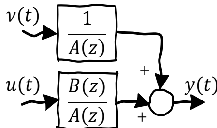
ARX
